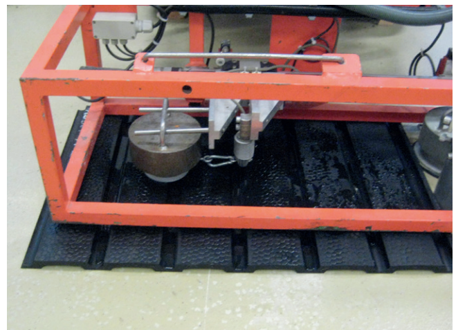
Bild 4: Messung der Rutschfestigkeit
