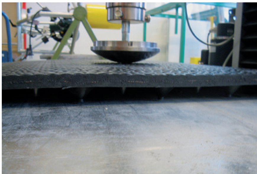
Bild 3: Messung der Verformbarkeit
