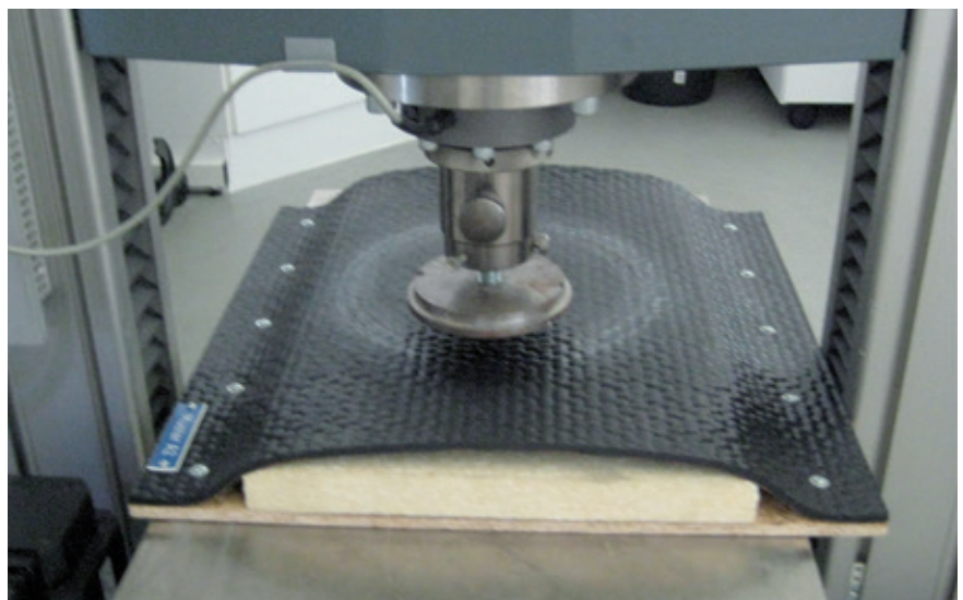
Bild 2: Messung der Verformbarkeit
