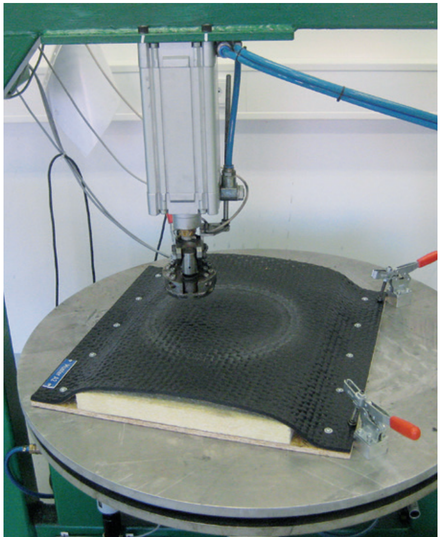
Bild 4: Dauertrittbelastung
