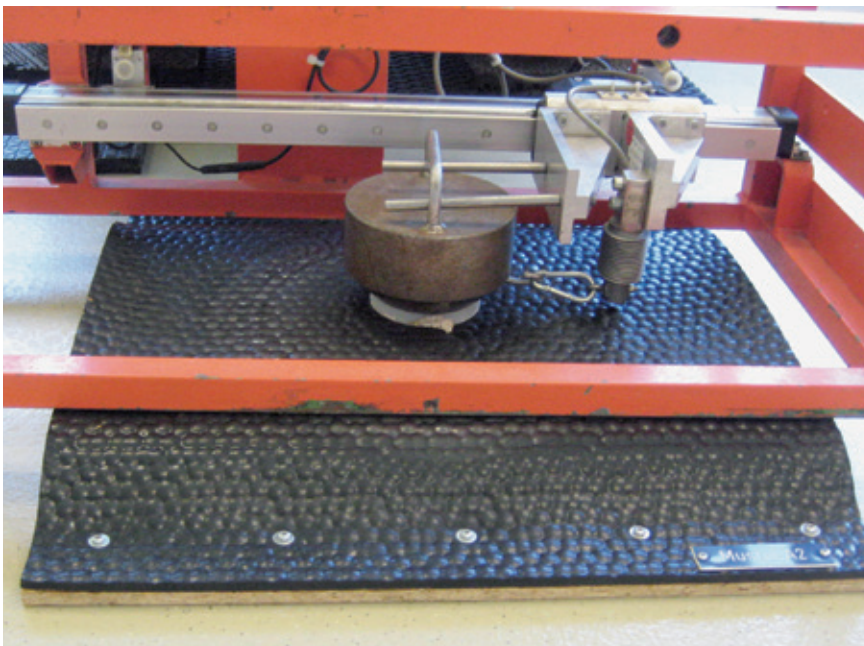
Bild 6: Messung der Rutschfestigkeit
