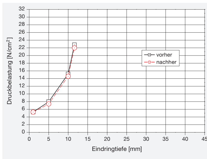
Bild 2: Verformbarkeit in Abhängigkeit vom Auflagedruck
